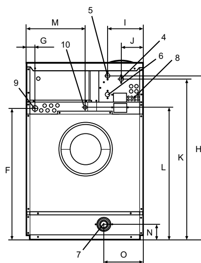
Arrière
